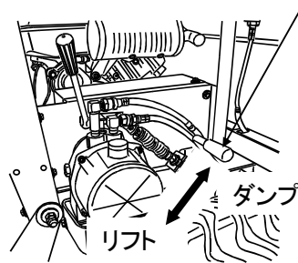
リフト・ダンプ切換レバー
